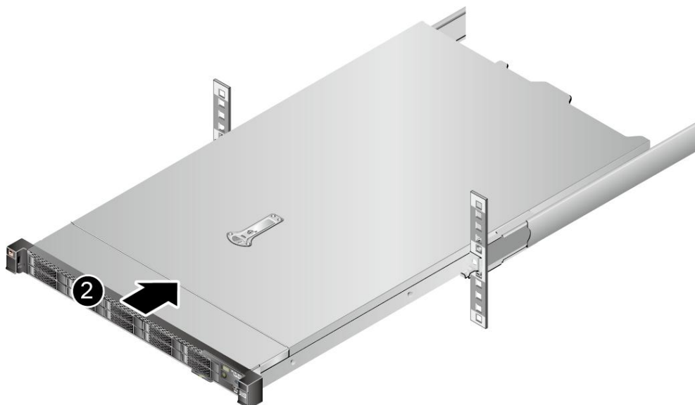
图 6-13 将服务器推入静态滑轨
