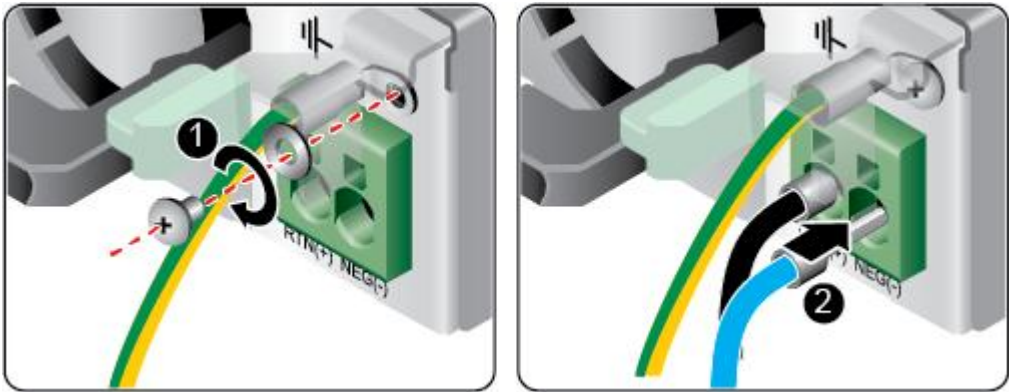
图 6-25 连接线缆
