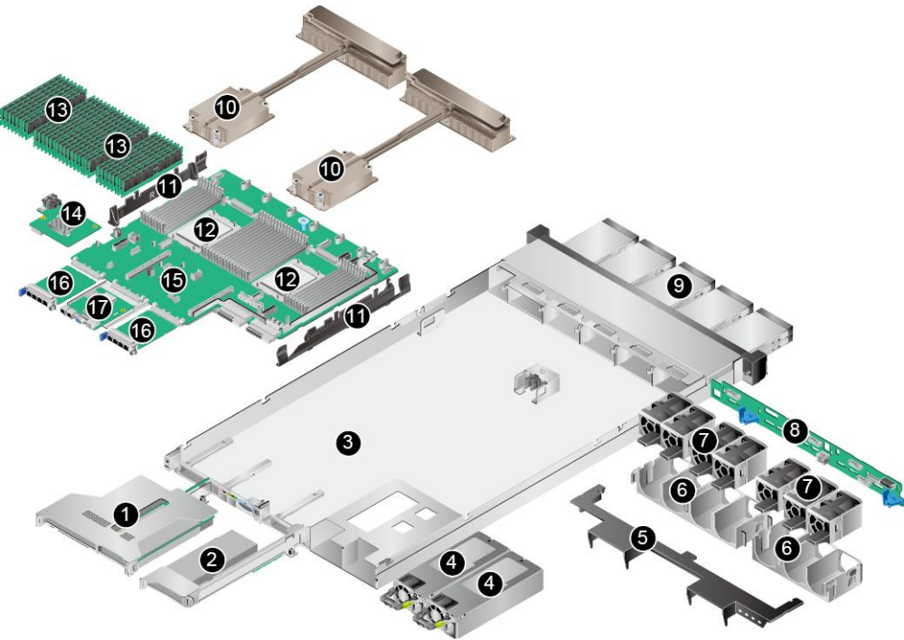
图 2-3 部件（配置异形散热器）
