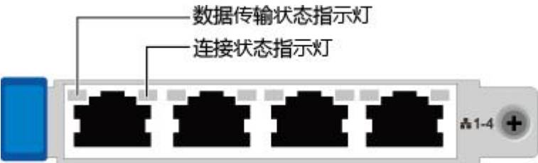
图 3-5 TM210（4*GE 电口）
