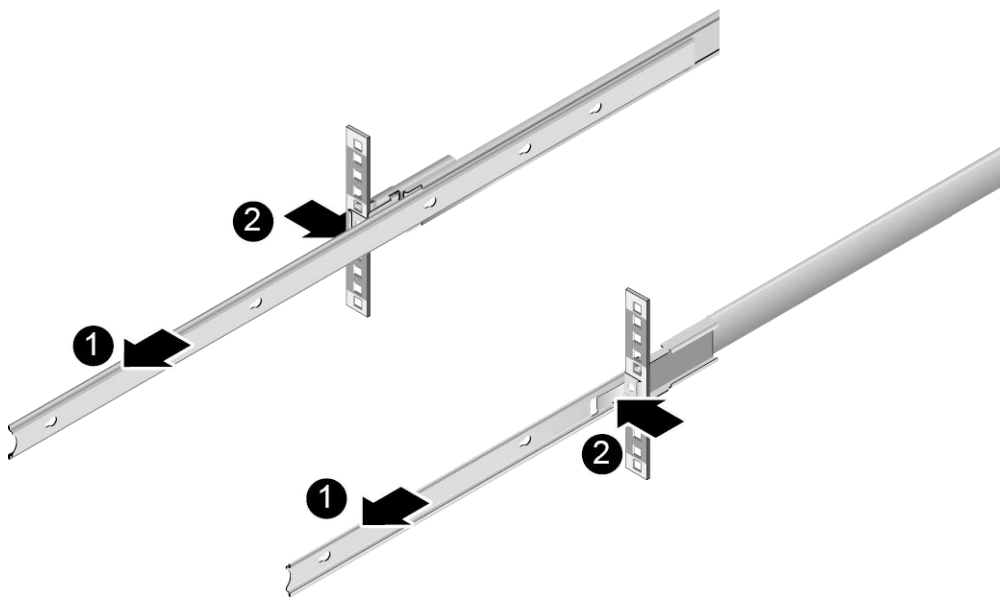
图 6-10 抽出内轨
