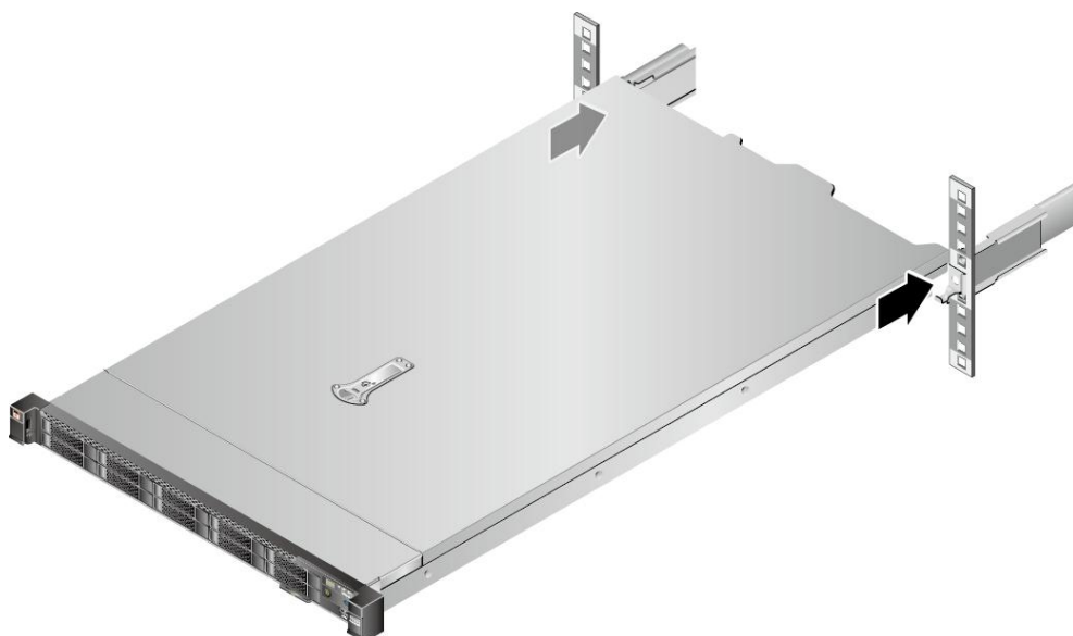
图 6-12 安装服务器
