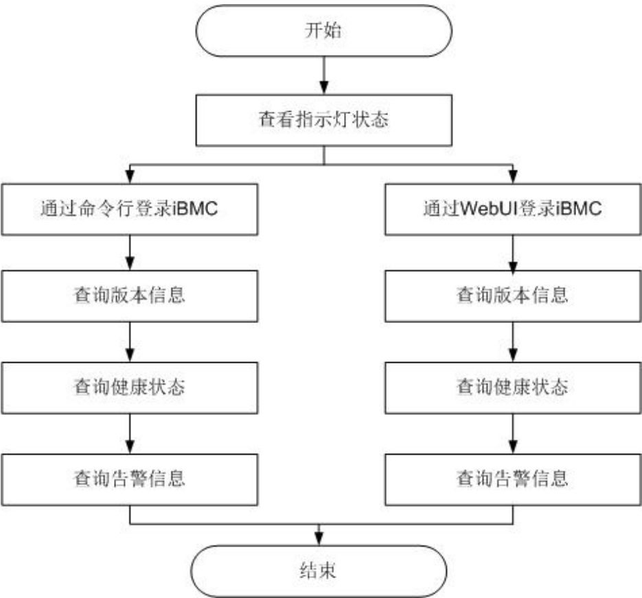
图 6-32 检查流程
