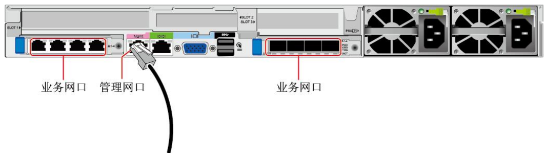
图 6-16 连接网线
