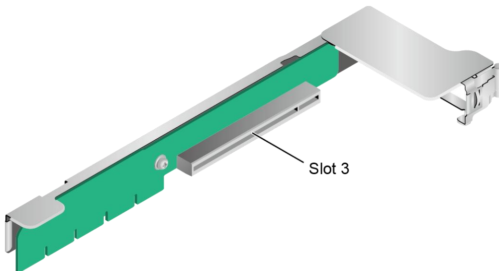
图 3-11 Riser 卡 2（Slot 3 x16）（板名：BC82PRUW）
