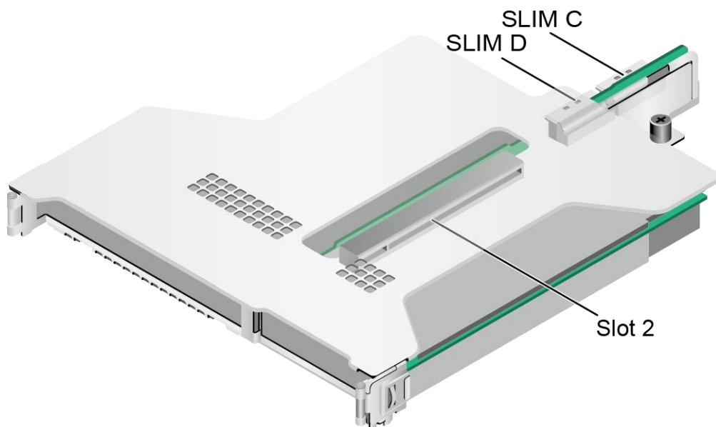
图 3-13 Riser 卡 4（Slot 2 x8）（板名：BC82PRUT）
