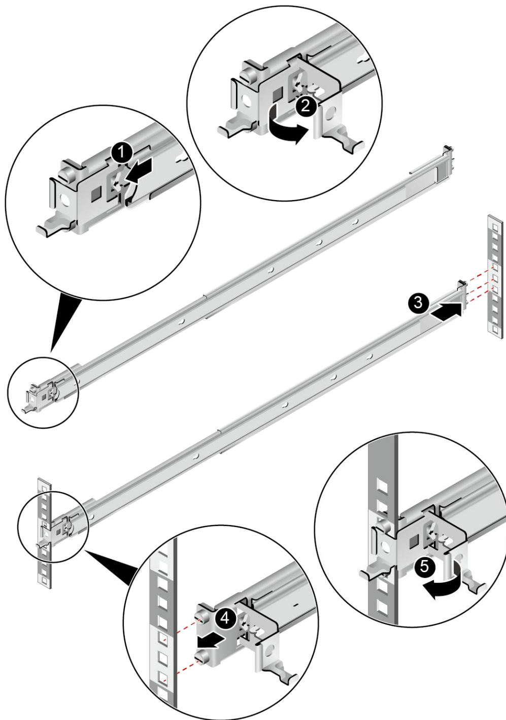
图 6-9 安装静态滑轨前后端
