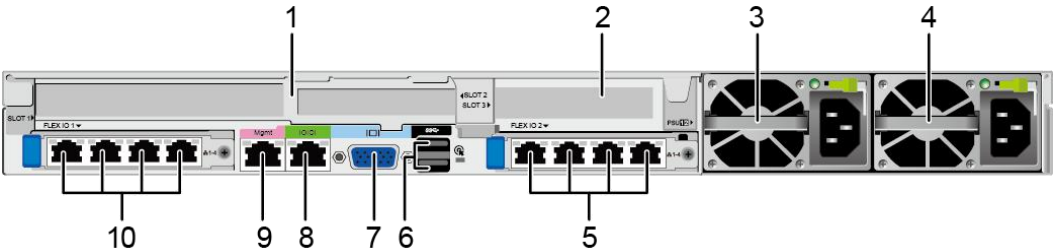
图 3-3 后面板组件
