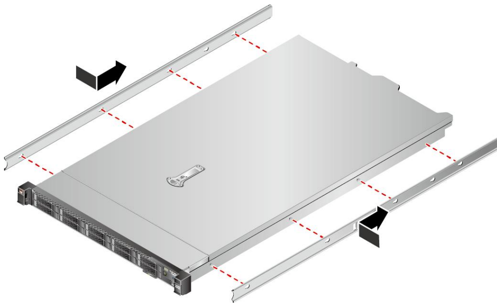
图 6-11 安装内轨到服务器
