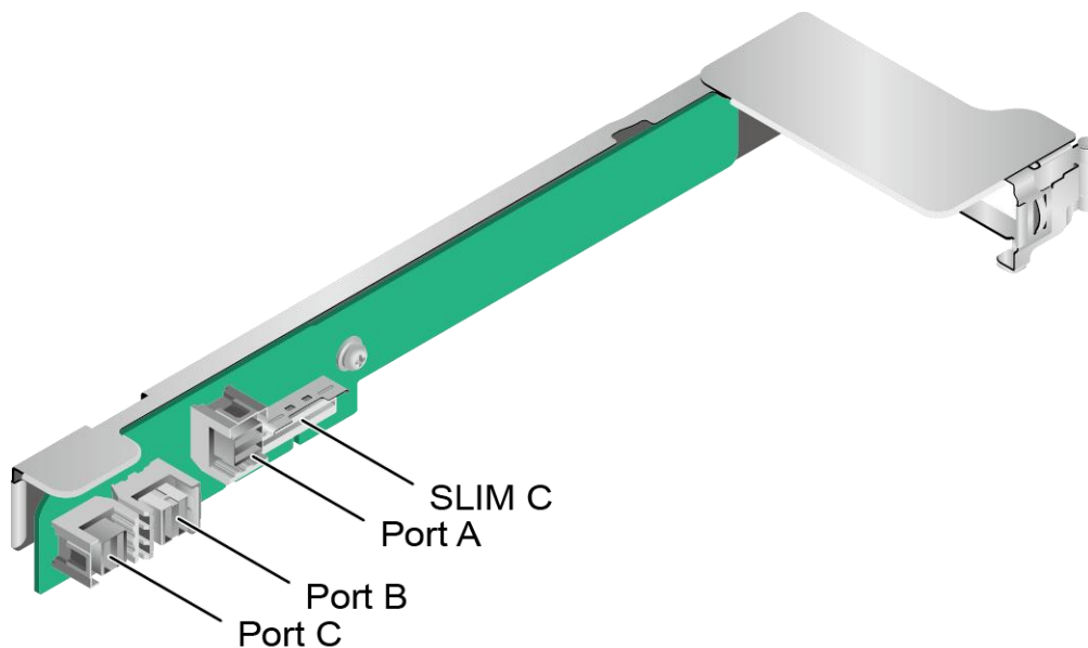
图 3-12 Riser 卡 3（板名：BC82PRUS）
