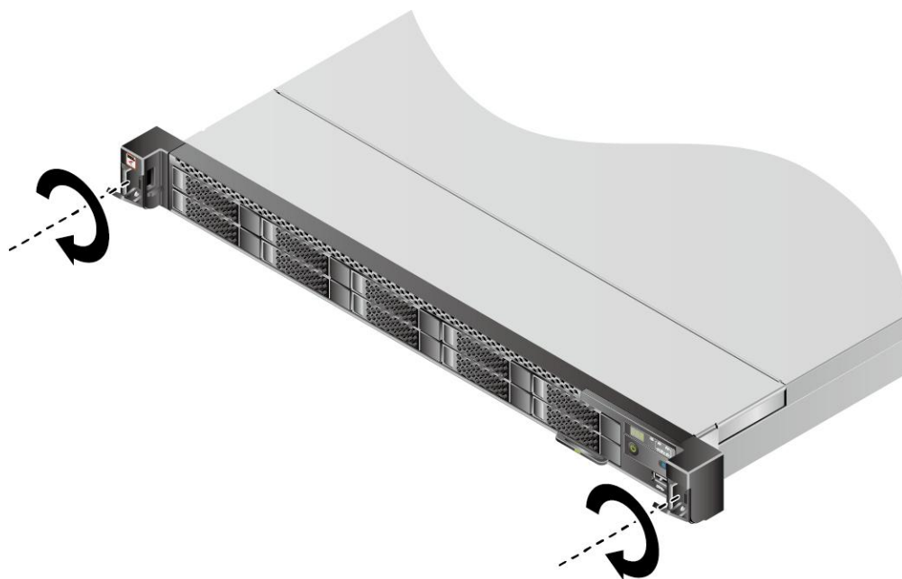
图 6-14 固定服务器
