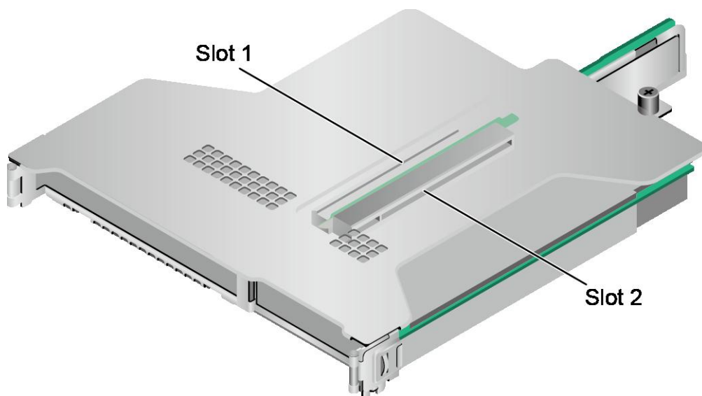
图 3-10 Riser 卡 1（Slot 1 x16+Slot 2 x8）（板名：BC82PRUV）
