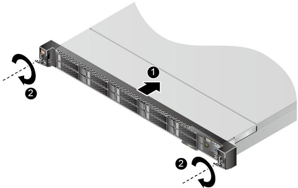
图 6-8 安装服务器
