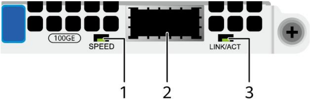
图 5-44 SF225S-H（1x100GE 光口）
