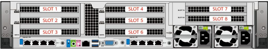
图 5-41 PCIe 插槽
