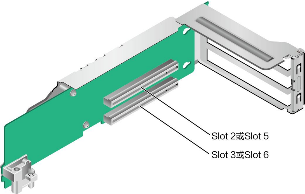
图 5-34 2*x8 Riser 卡
