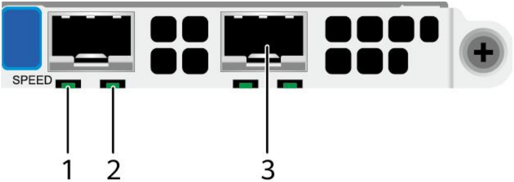
图 5-43 SF223D-H（2x25GE 光口）
