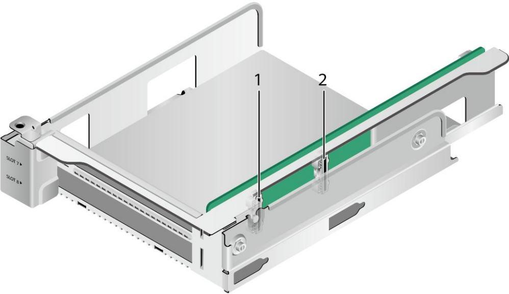
图 5-38 2*x8 Riser 卡（反面）
