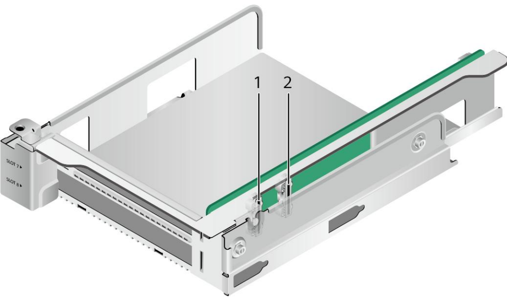
图 5-40 1*x16 Riser 卡（反面）
