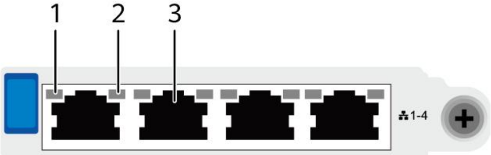
图 5-42 SF221Q（4xGE 电口）
