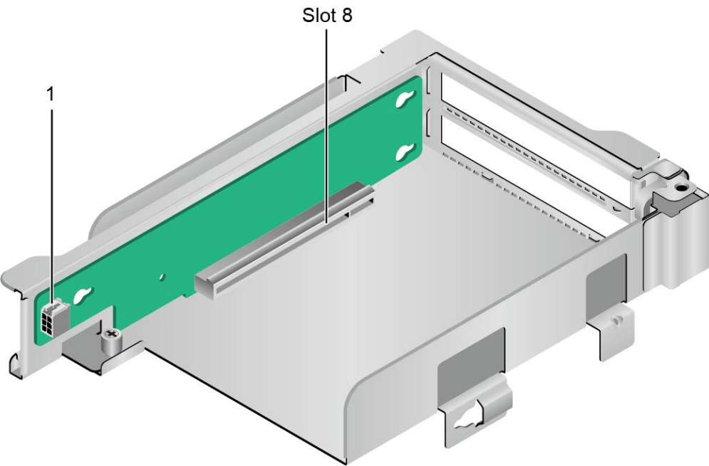
图 5-39 1*x16 Riser 卡（正面）
