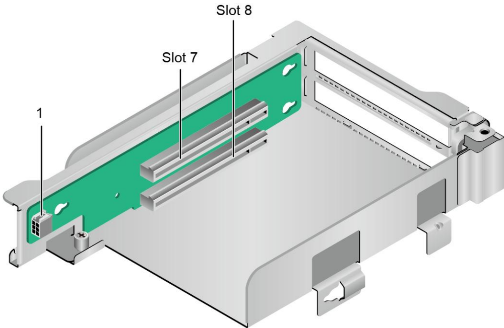
图 5-37 2*x8 Riser 卡（正面）
