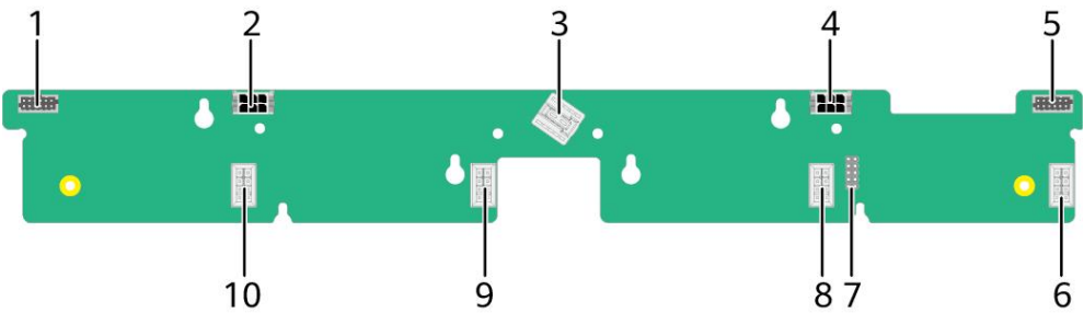
图 5-9 风扇板接口
