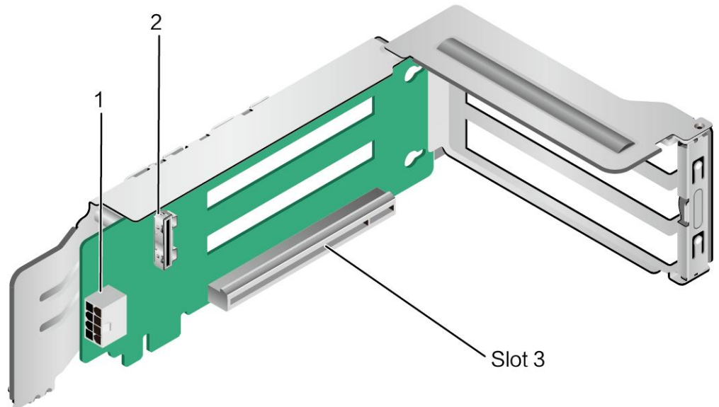
图 5-36 1*x8 Riser 卡（正面）
