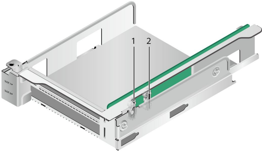
图 5-28 1*x16 Riser 卡（反面）
