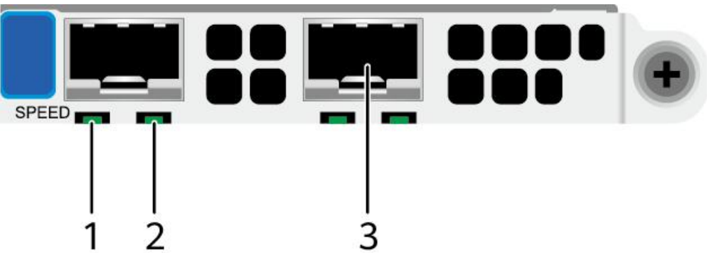
图 5-31 SF223D-H（2x25GE 光口）
