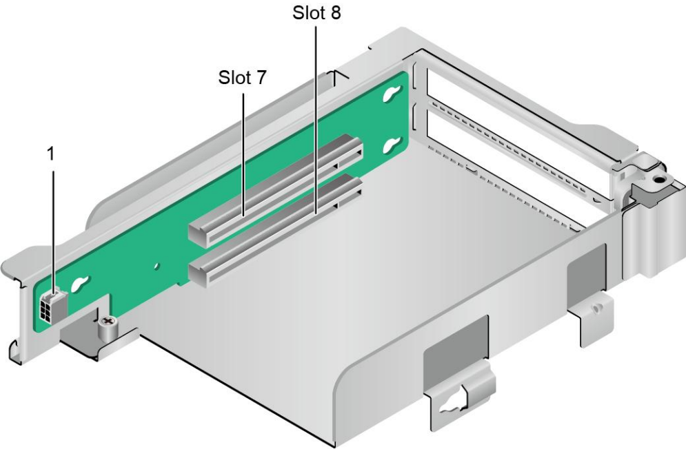
图 5-25 2*x8 Riser 卡（正面）
