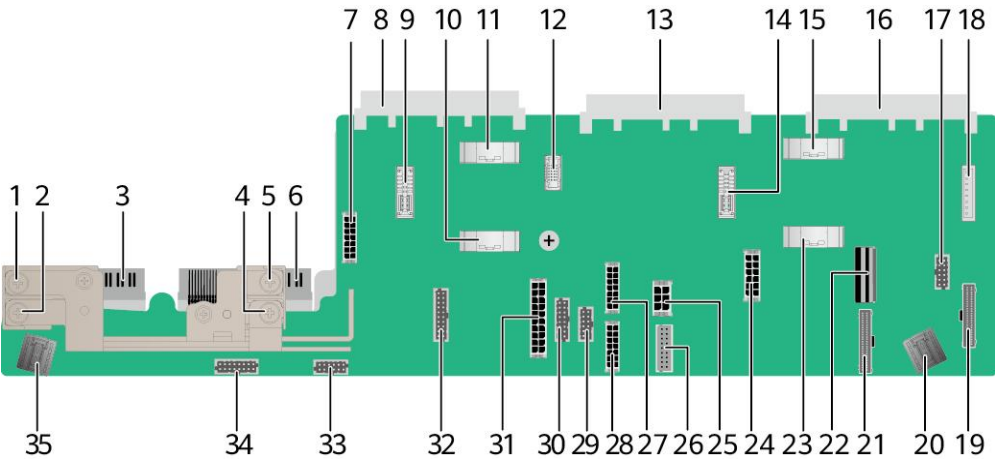
图 5-5 扩展板
