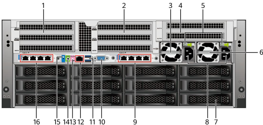
图 5-2 后面板
