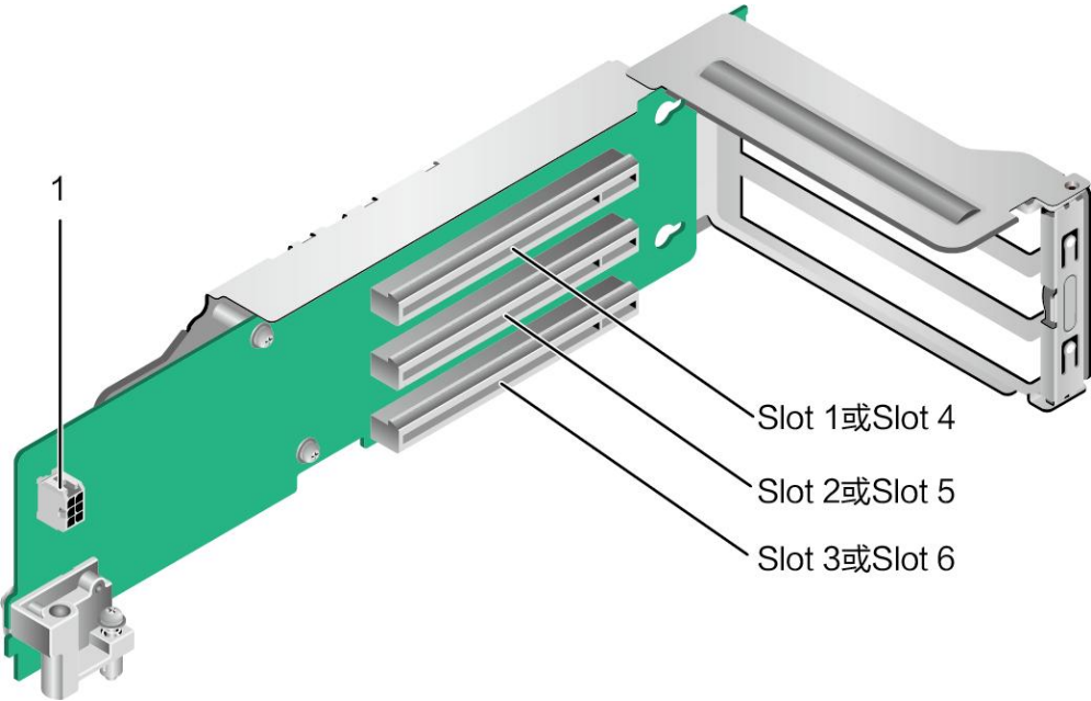
图 5-21 3*x8 Riser 卡（正面）
