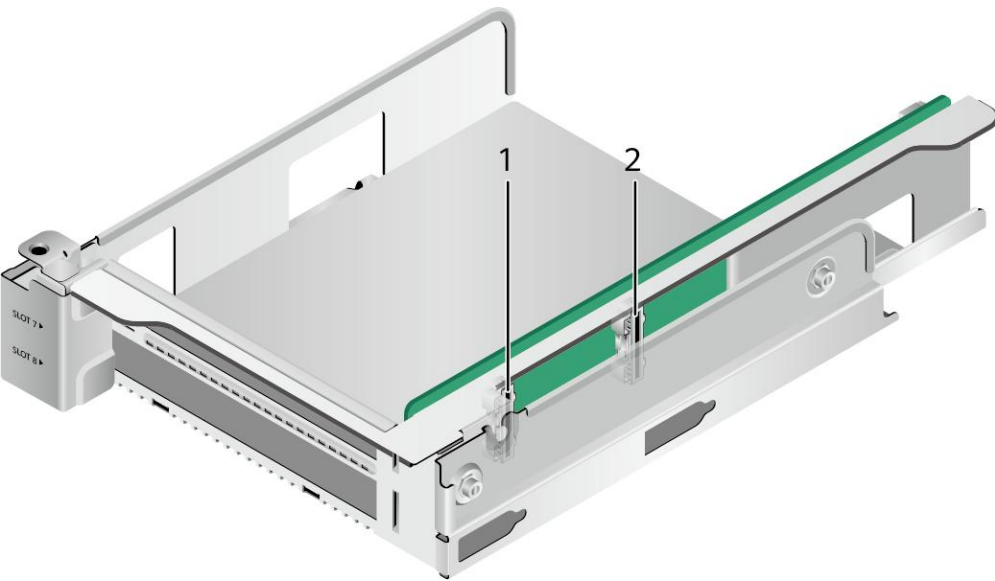
图 5-26 2*x8 Riser 卡（反面）
