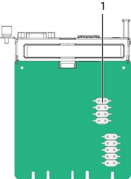
图 5-33 BMC 插卡
