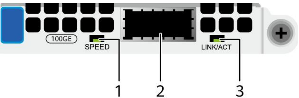
图 5-32 SF225S-H（1x100GE 光口）
