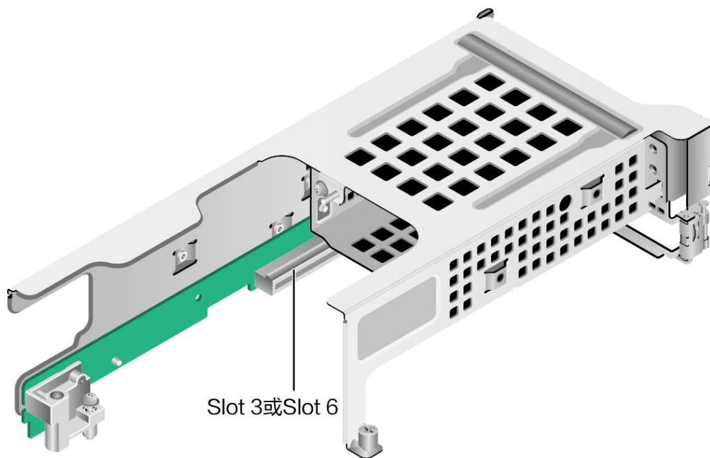
图 5-24 1*x16 Riser 卡
