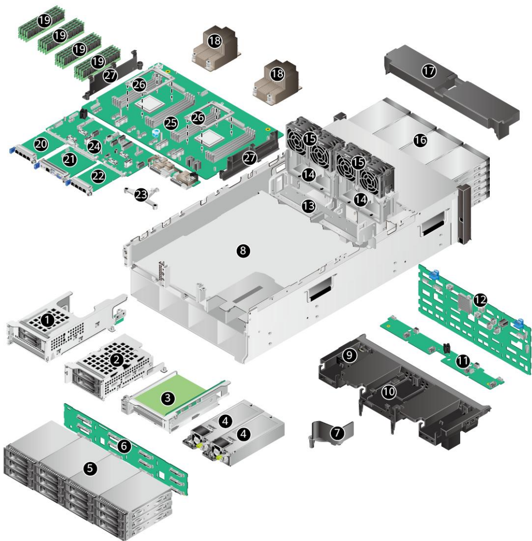
图 3-1 部件
