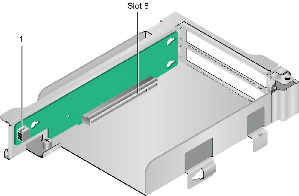
图 5-27 1*x16 Riser 卡（正面）
