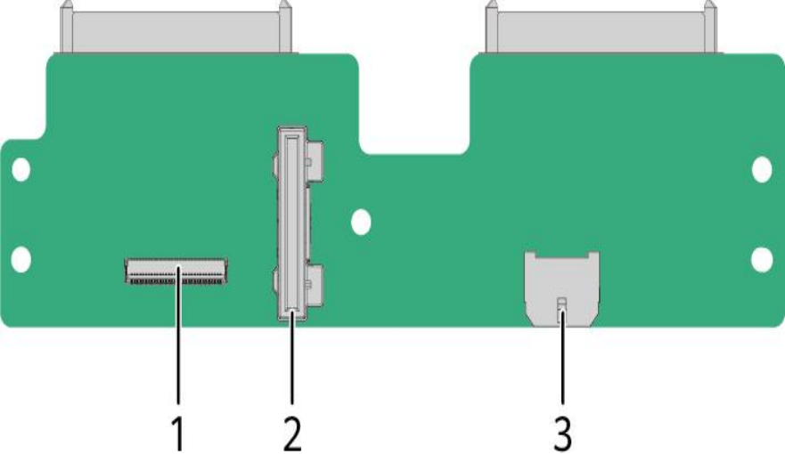
图 5-19 IO 模组 3 水平硬盘背板（上板）
