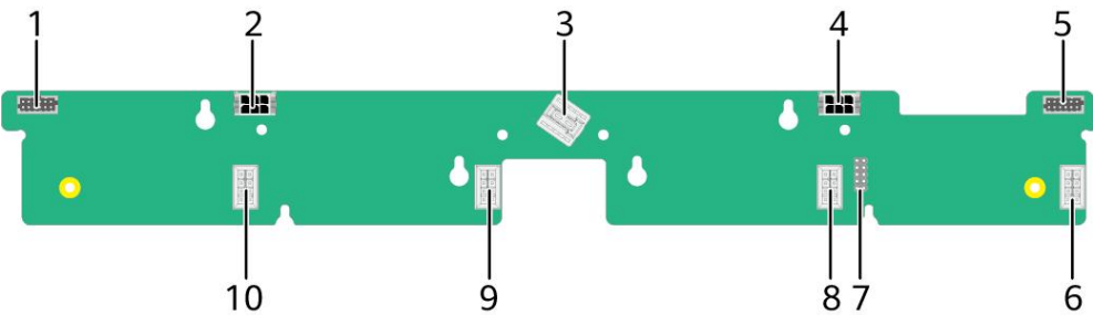
图 5-6 风扇板接口
