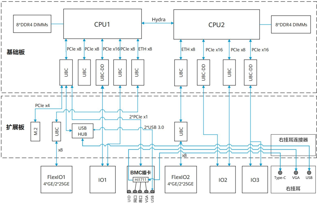
图 4-1 逻辑结构
