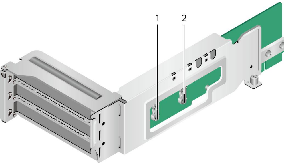
图 5-22 3*x8 Riser 卡（反面）
