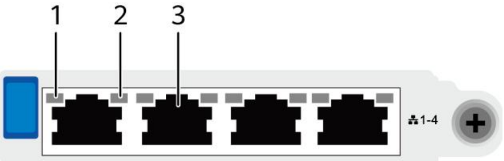
图 5-30 SF221Q（4xGE 电口）
