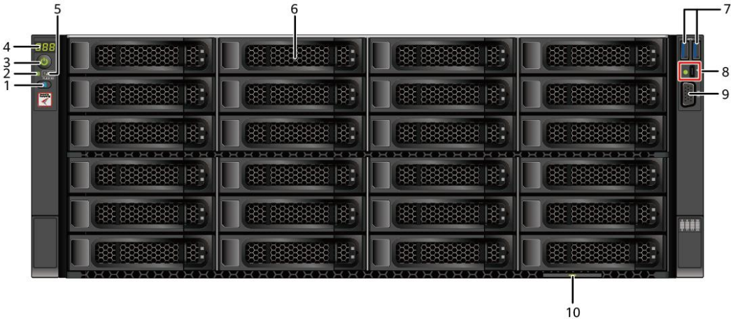
图 5-1 36x3.5 英寸硬盘配置前面板
