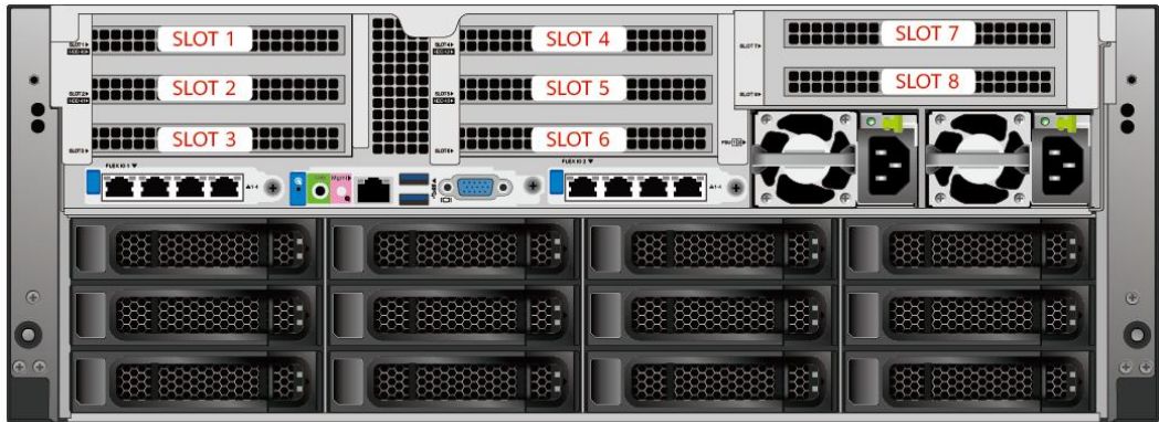
图 5-29 PCIe 插槽
