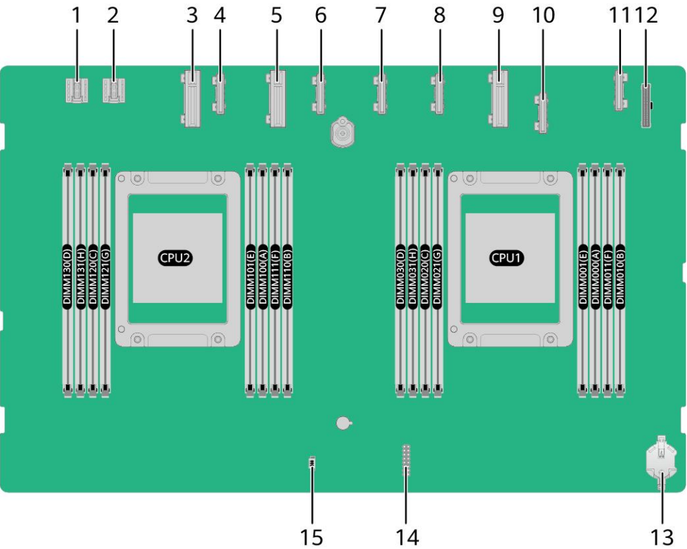
图 5-3 基础板接口
